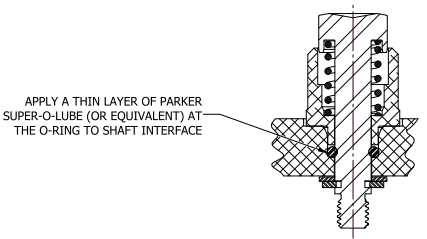
BUTTON INSTALL SCALE 4 : 1
